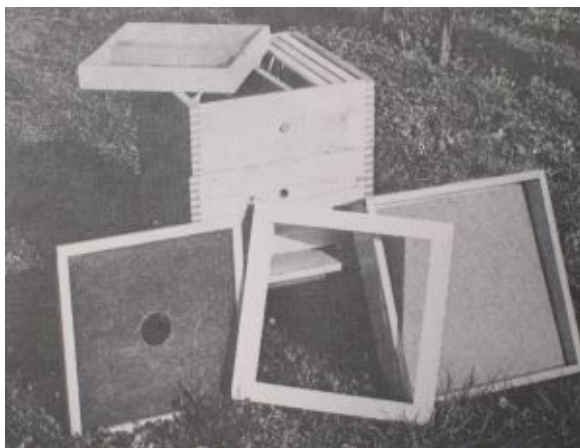
Části úlu - dva nízké nástavky a krmítko, vpředu přepážka, polystyrénový límec ke krmítku, vnější kryt (víko)
