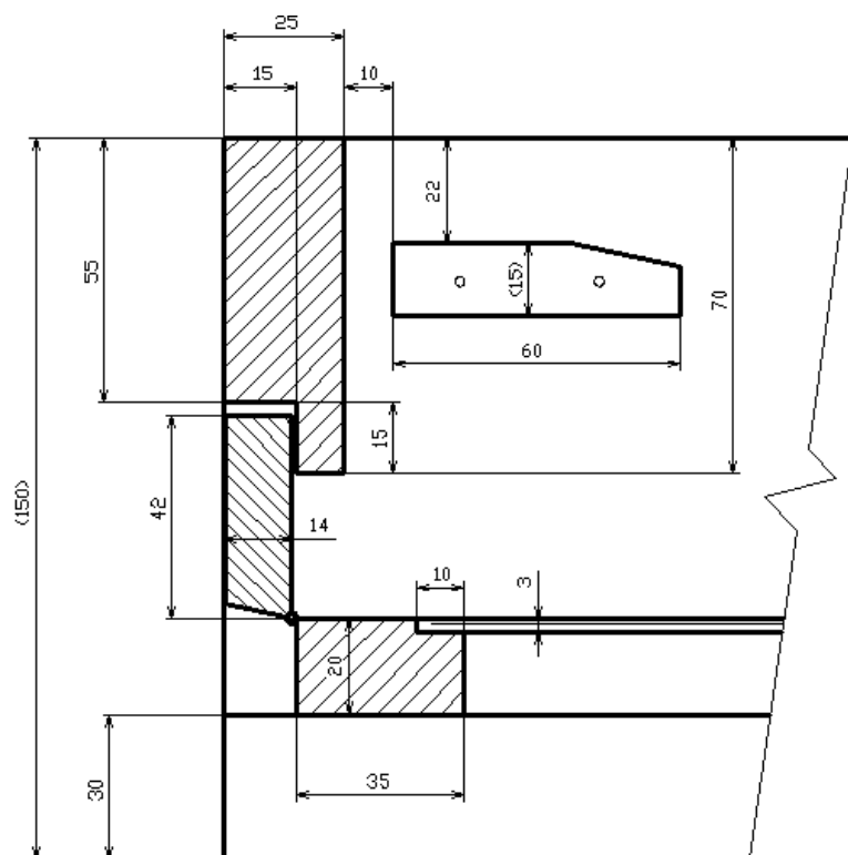
Obr. 4 Řez - přední část
