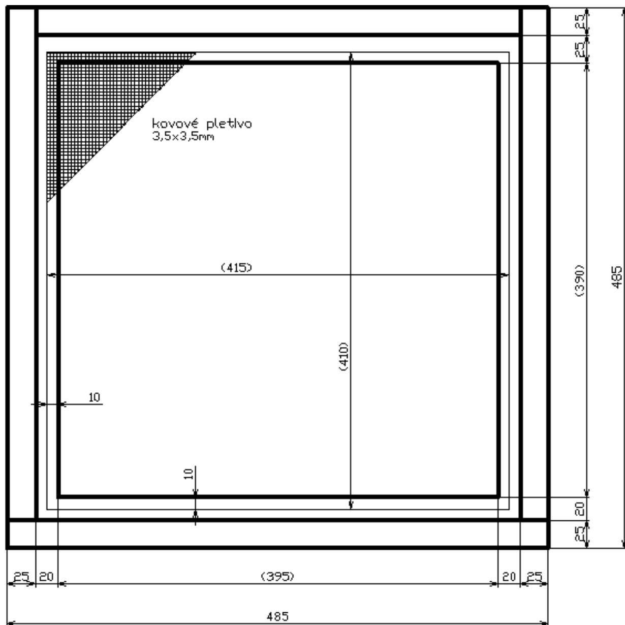
Obr. 3 Pohled shora
