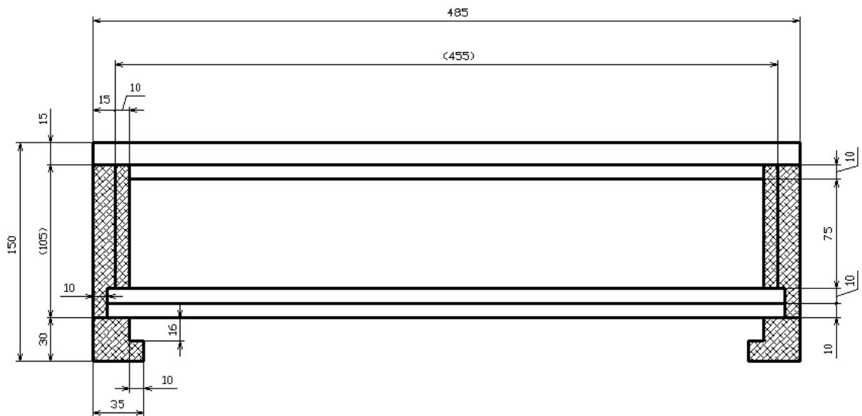
Obr. 2 Pohled zezadu (bez zadního víčka)
